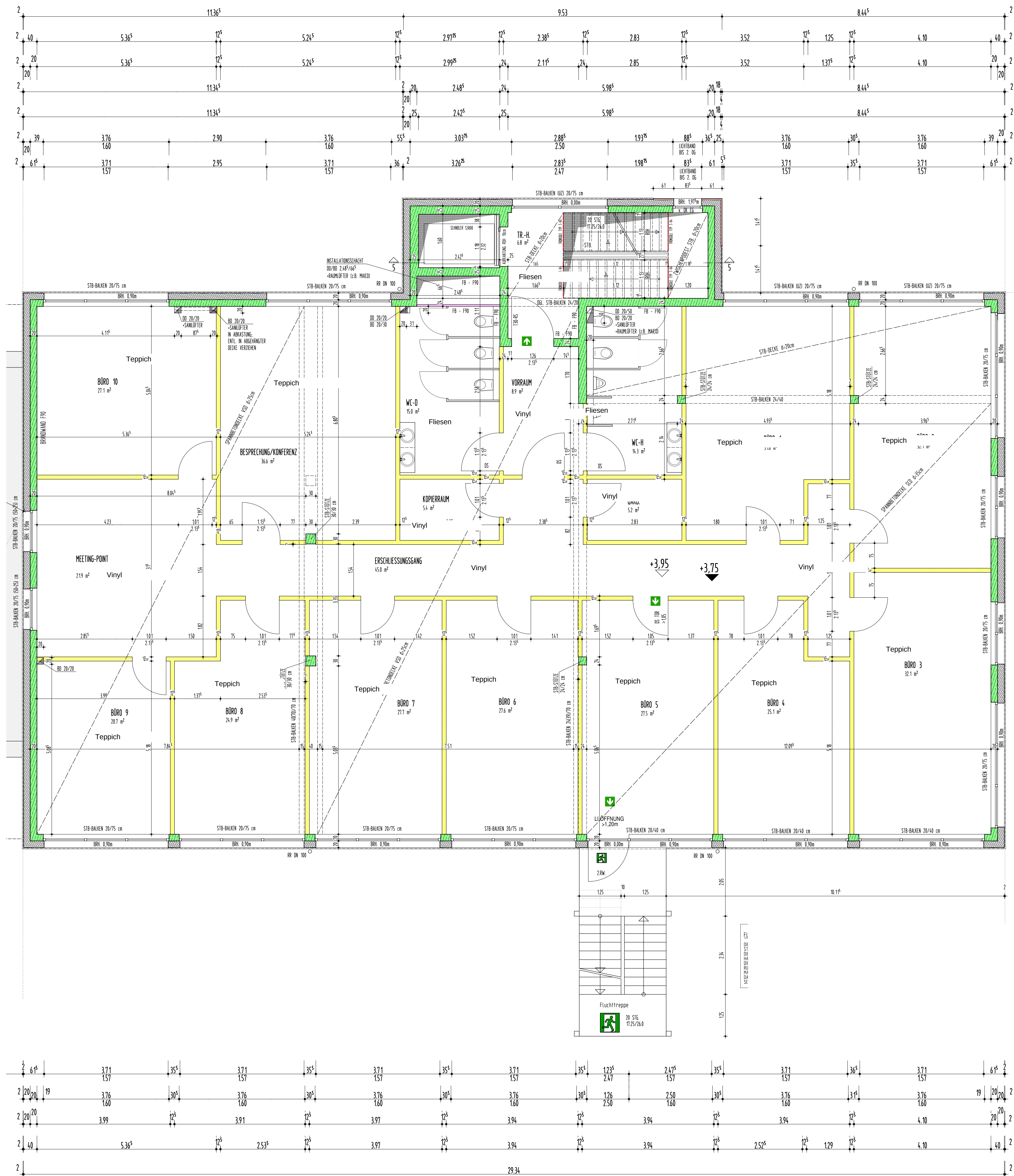
1. OBERGESCHOSS -AUFSTOCKUNG-
